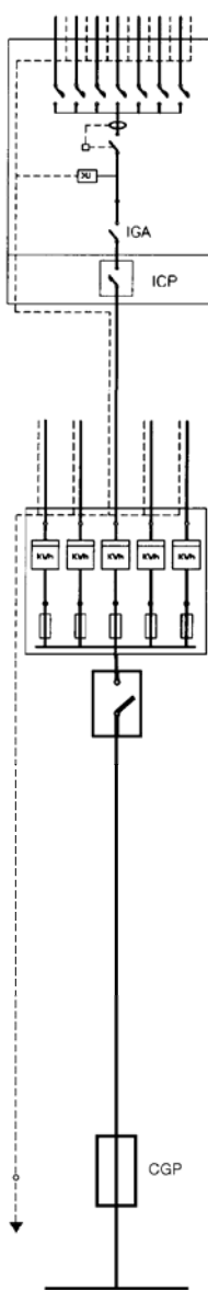
ESQUEMA UNIFILAR
