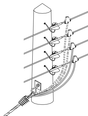
DETALL "B"
