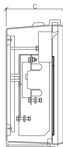
SECCIÓ B-B'
