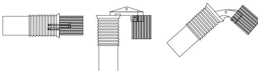
Figura 3. Frontissa rígida
