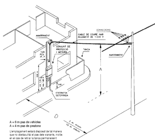
DETALLS D'INSTAL·LACIÓ
