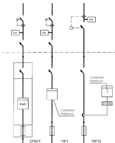
ESQUEMES UNIFILARS
